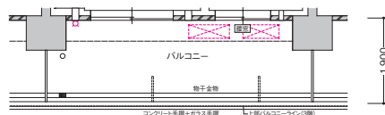
2.3階部分図 scale:約1/150
