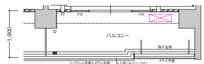
3階部分図 scale:約1/150
