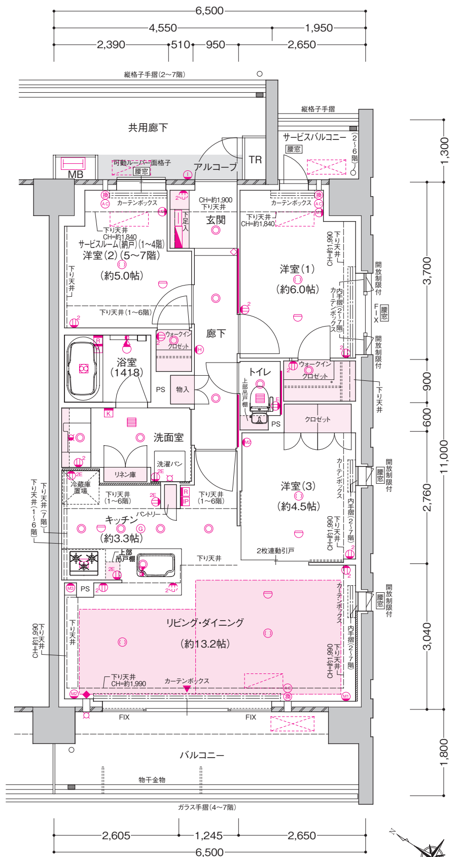
2階部分図 scale:約1/150
