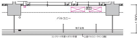
■ 2・3階部分図 scale:約1/150
