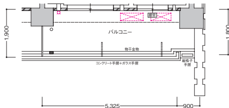
2階部分図 scale:約1/150
