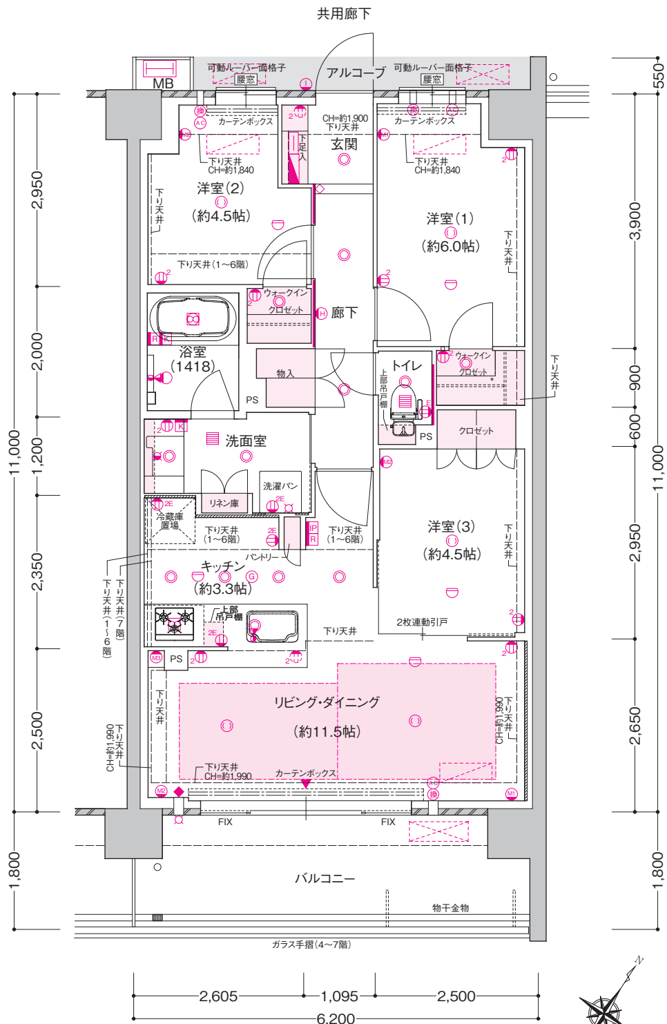
2階部分図 scale:約1/150
