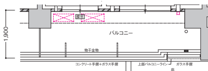
2階部分図 scale:約1/150
